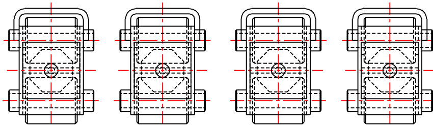
4-5000 LBS.(2.5 TON) CS-3H SWIVEL TOP SKATES
